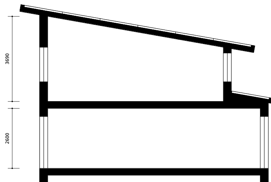
Principeddoorsnede
