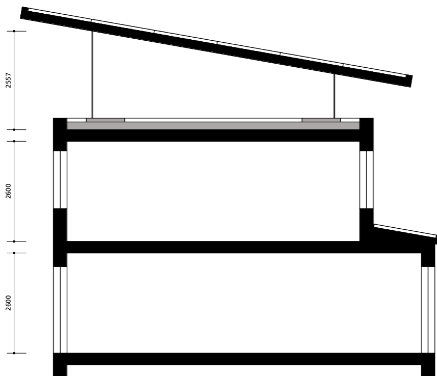
Principedoorsnede
